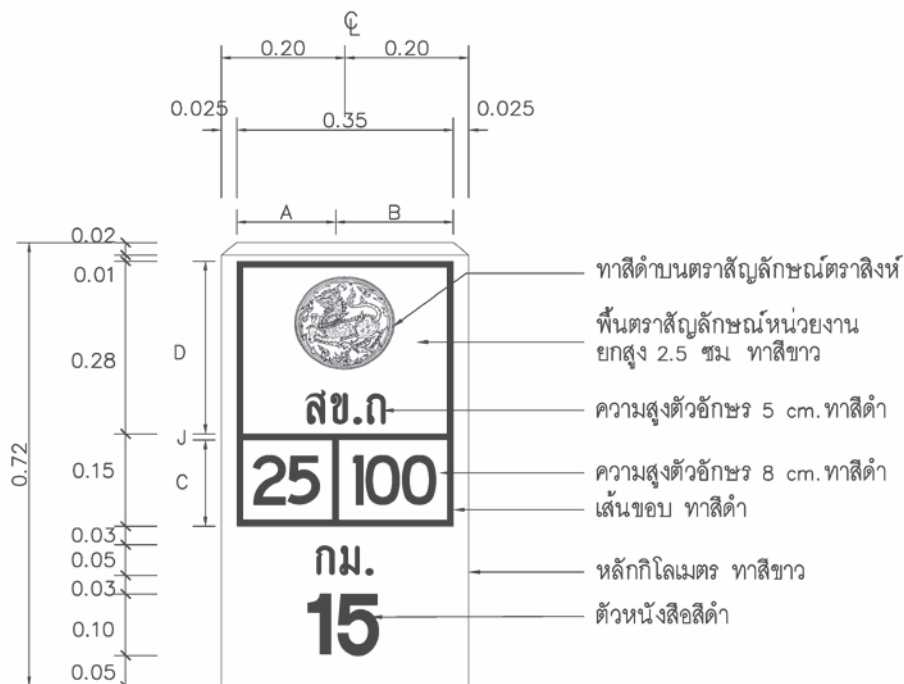
รูปที่ ข-๑๐ ตัวอย่างและรายละเอียดหลักกิโลเมตร
