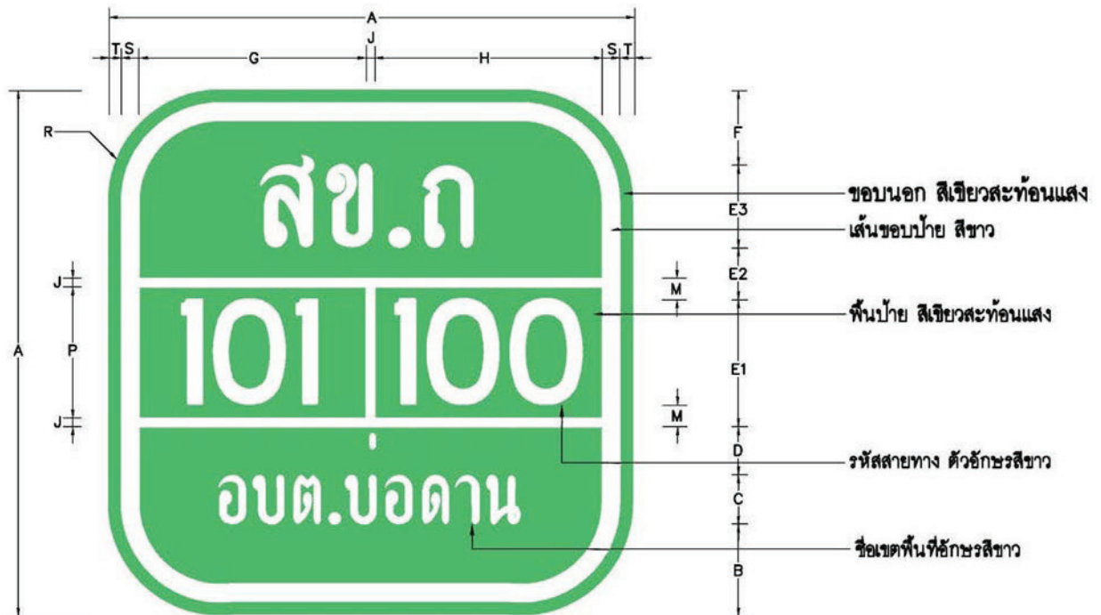
รูปที่ ข-๙ ตัวอย่างและรายละเอียดป้ายหมายเลขทางหลวงท้องถิ่น (น-๑/๑) ขนาด ๗๕x๗๕ ซม. (สำหรับ อบท. ลำดับที่ ๑๐๐- ๙๙๙)
