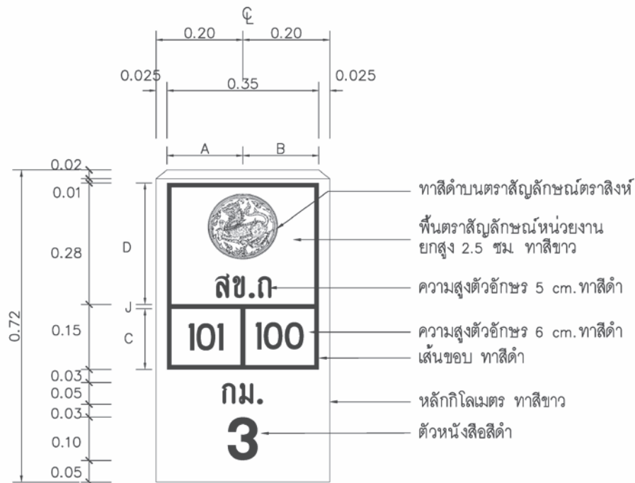
รูปที่ ข-๑๑ ตัวอย่างและรายละเอียดหลักกิโลเมตร สำหรับ อปท. ลำดับที่ ๑๐๐ - ๙๙๙ และมีลำดับของสายทางตั้งแต่ ๑๐๐ - ๙๙๙
