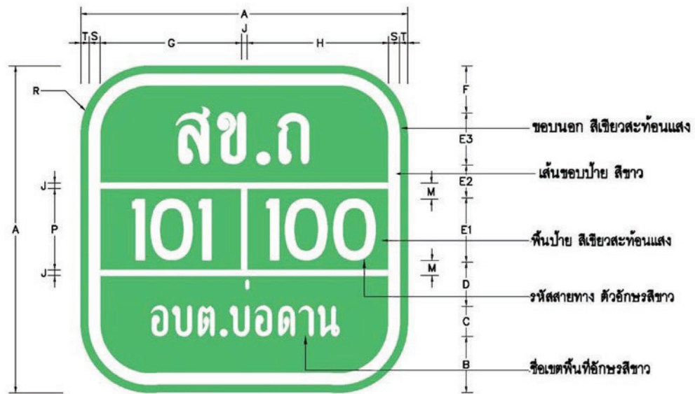
รูปที่ ข-๘ ตัวอย่างและรายละเอียดป้ายหมายเลขทางหลวงท้องถิ่น (น-๑/๑) ขนาด ๖๐x๖๐ ซม. (สำหรับ อบท. ลำดับที่ ๑๐๐ - ๙๙๙)
